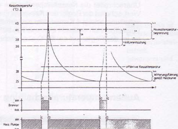
Witterungsgeführte Minimaltemperaturbegrenzung mit Anfahrntlastung.
